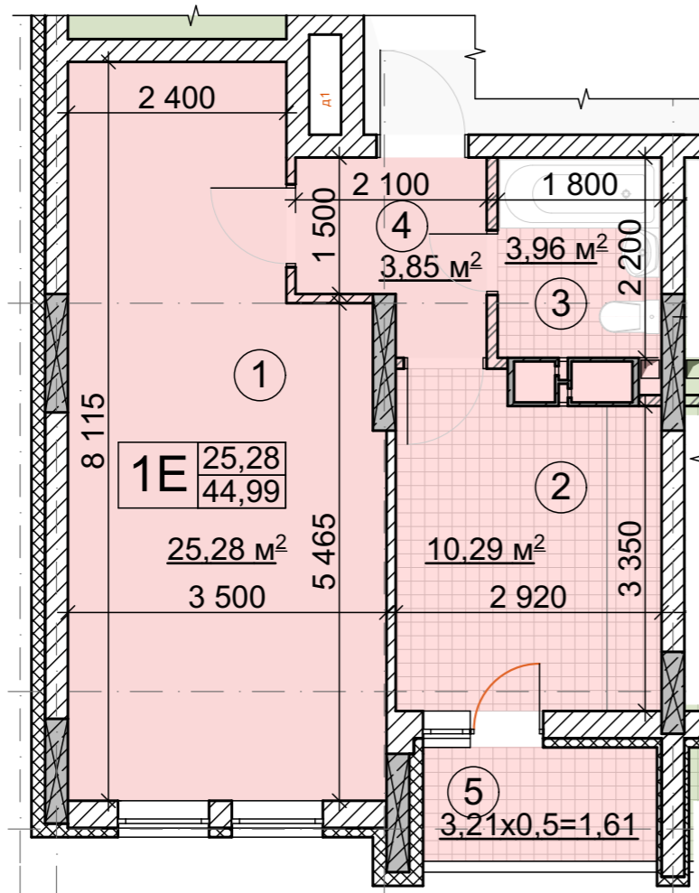
Схема розташування квартири на поверсі
